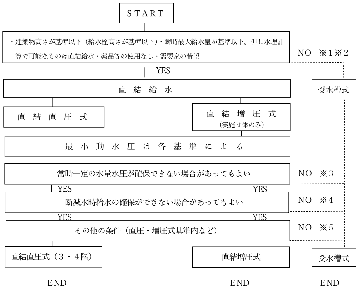
給水形態の選定フロー
