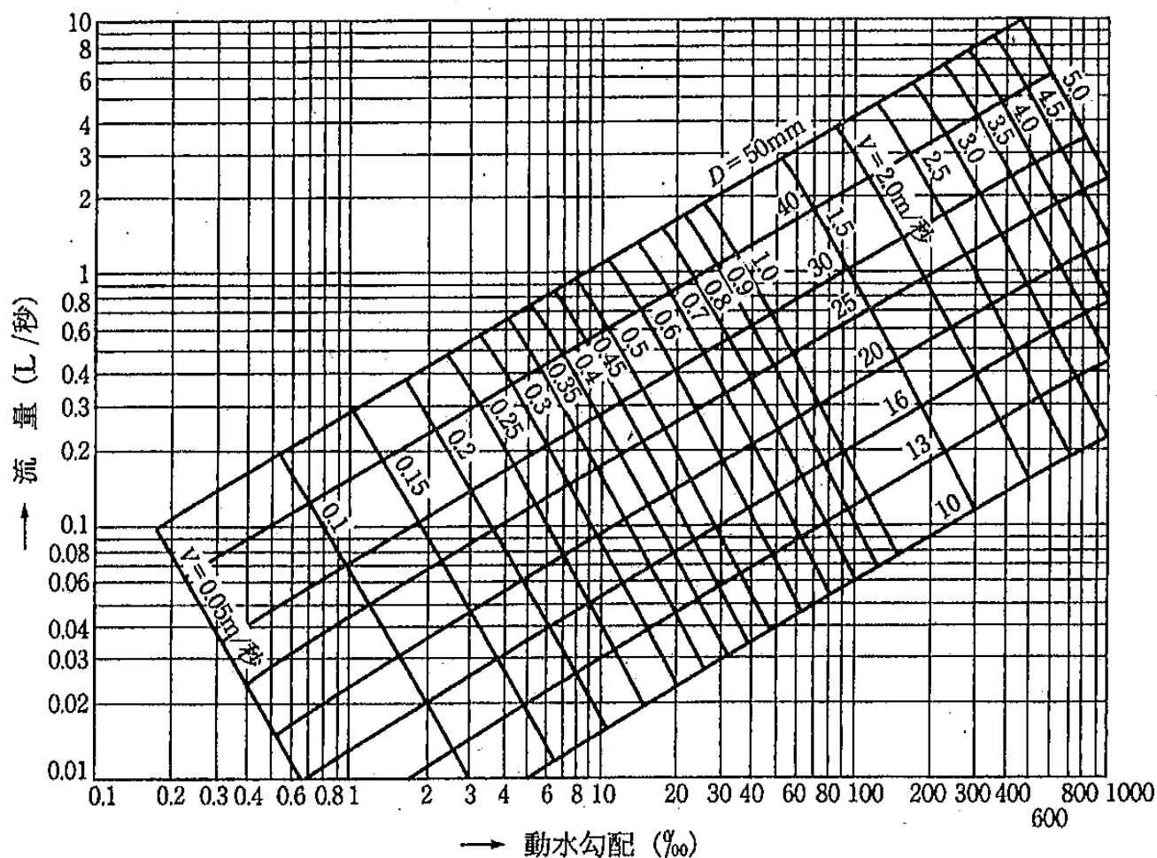
図 3.5.2 ウェストン公式流量図
