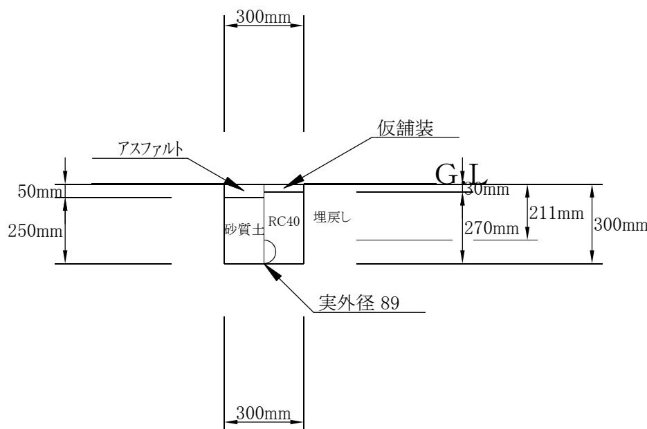
土工①VLG φ75 布設（掘削・埋戻し） 1／20
