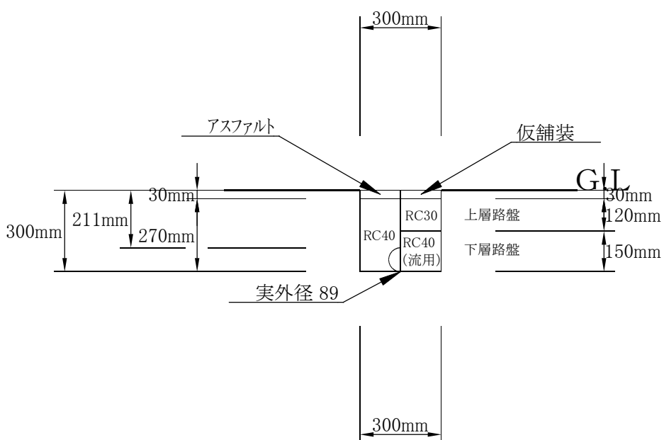
土工②VLG φ75 撤去（掘削・埋戻し） 1／20
