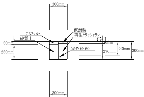
② VLGφ50布設（掘削・埋戻し） 1/20
