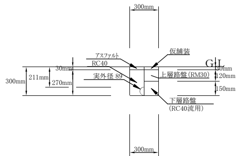
① VLGφ75撤去（掘削・埋戻し） 1/20
