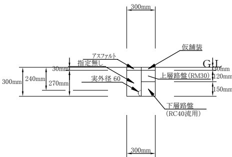
② VLGφ50撤去（掘削・埋戻し） 1/20
