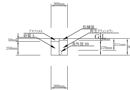
①土工 VLGφ75布設（掘削・埋戻し） 1/20
