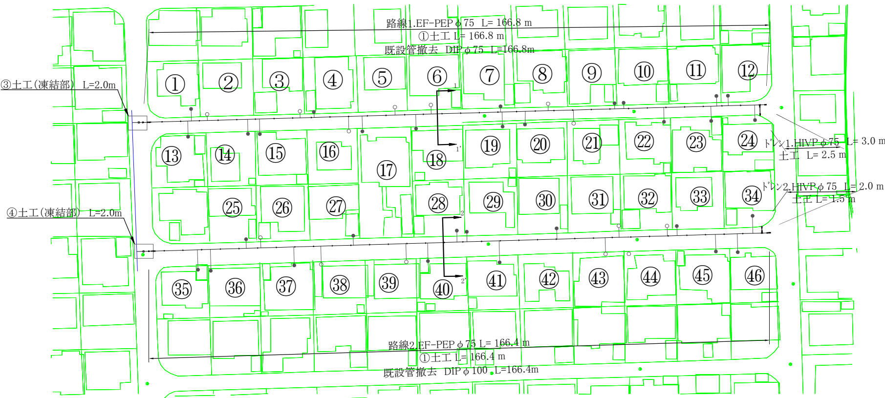
配管詳細図 S = No Scale
