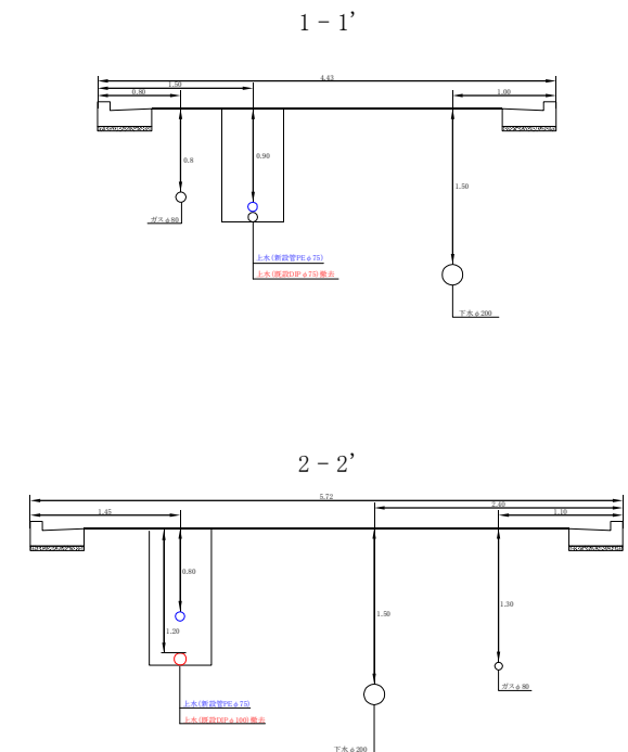
横断面図 S = 1 : 40
