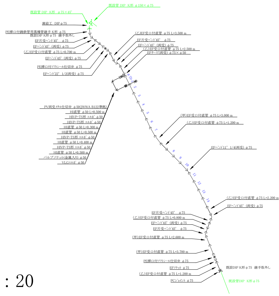
①土工 EF-PEPφ75 (掘削・埋戻し) 1/20 (ガス工事跡施工部) ②土工 EF-PEPφ75 (掘削・埋戻し) 1/20 (水道単独部) トーンHVPφ50 (掘削・埋戻し) 1/20
