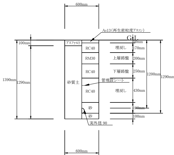
01: 車道EF-PEPφ75（掘削・埋戻し） 1/20
