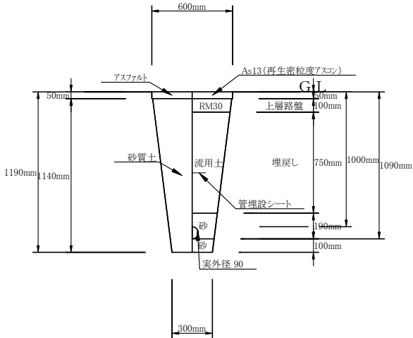
01': 歩道EF-PEPφ75（掘削・埋戻し） 1/20
