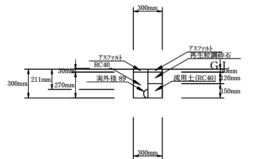
①土工 VLG φ75撤去（掘削・埋戻し） 1/20
