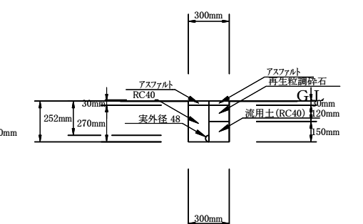
②土工 PE φ40撤去（掘削・埋戻し） 1/20
