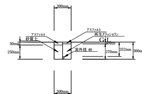
②土工 PE φ40布設（掘削・埋戻し） 1/20
