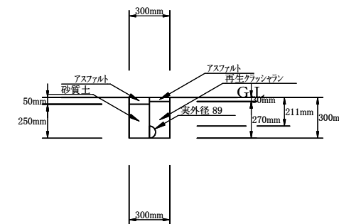
①土工 VLG φ75布設（掘削・埋戻し） 1/20
