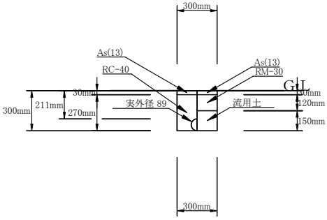
02:仮設 そのA 02: VLGφ75 撤去（掘削・埋戻し） 1／20
