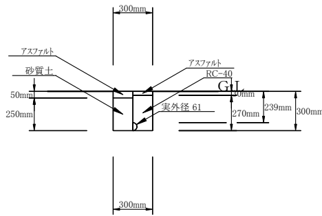
02:仮設 そのA 03: VLGφ50 布設（掘削・埋戻し） 1／20
