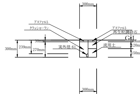
02:仮設 そのA 04: VLGφ50 撤去（掘削・埋戻し） 1／20
