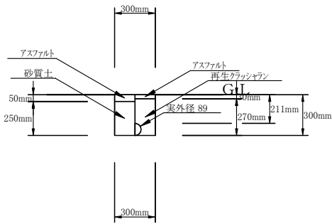
02:仮設 そのA 01: VLGφ75 布設（掘削・埋戻し） 1／20
