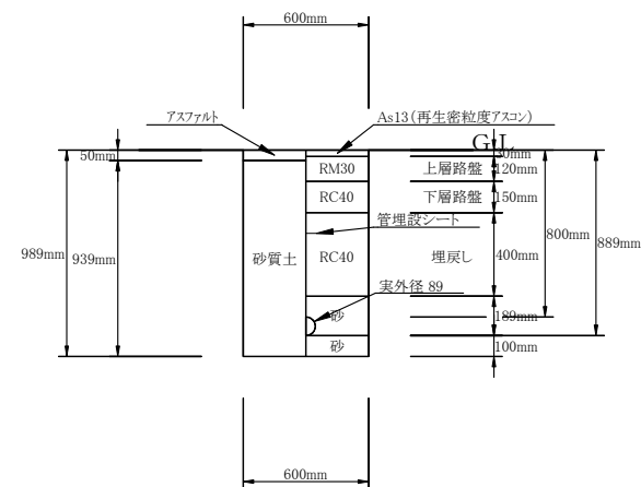
05:本設 そのA 02:トレンHVPφ75 (掘削・埋戻し) 1/20
