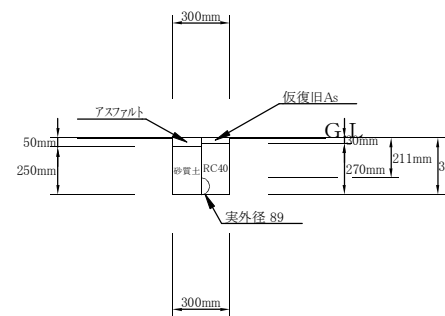
①土工(路線1、2) 仮設VLGφ75埋設 (掘削・埋戻し) 1/20
