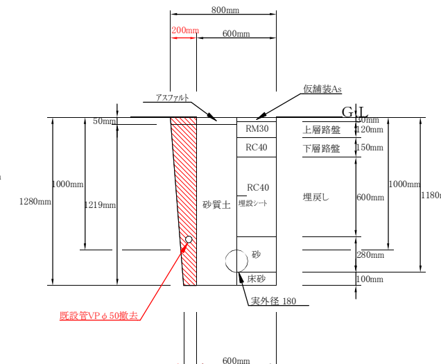
⑥ 土工(路線1-1) 既設管VPφ50 撤去部分(掘削・埋戻し) 1/20
