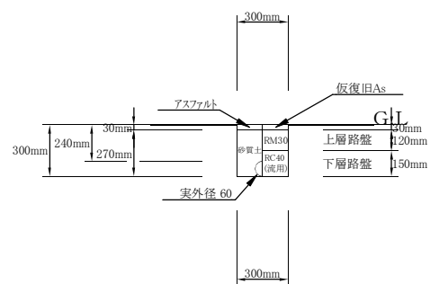
②土工(路線3、既設連絡1) 仮設VLGφ50撤去 (掘削・埋戻し) 1/20
