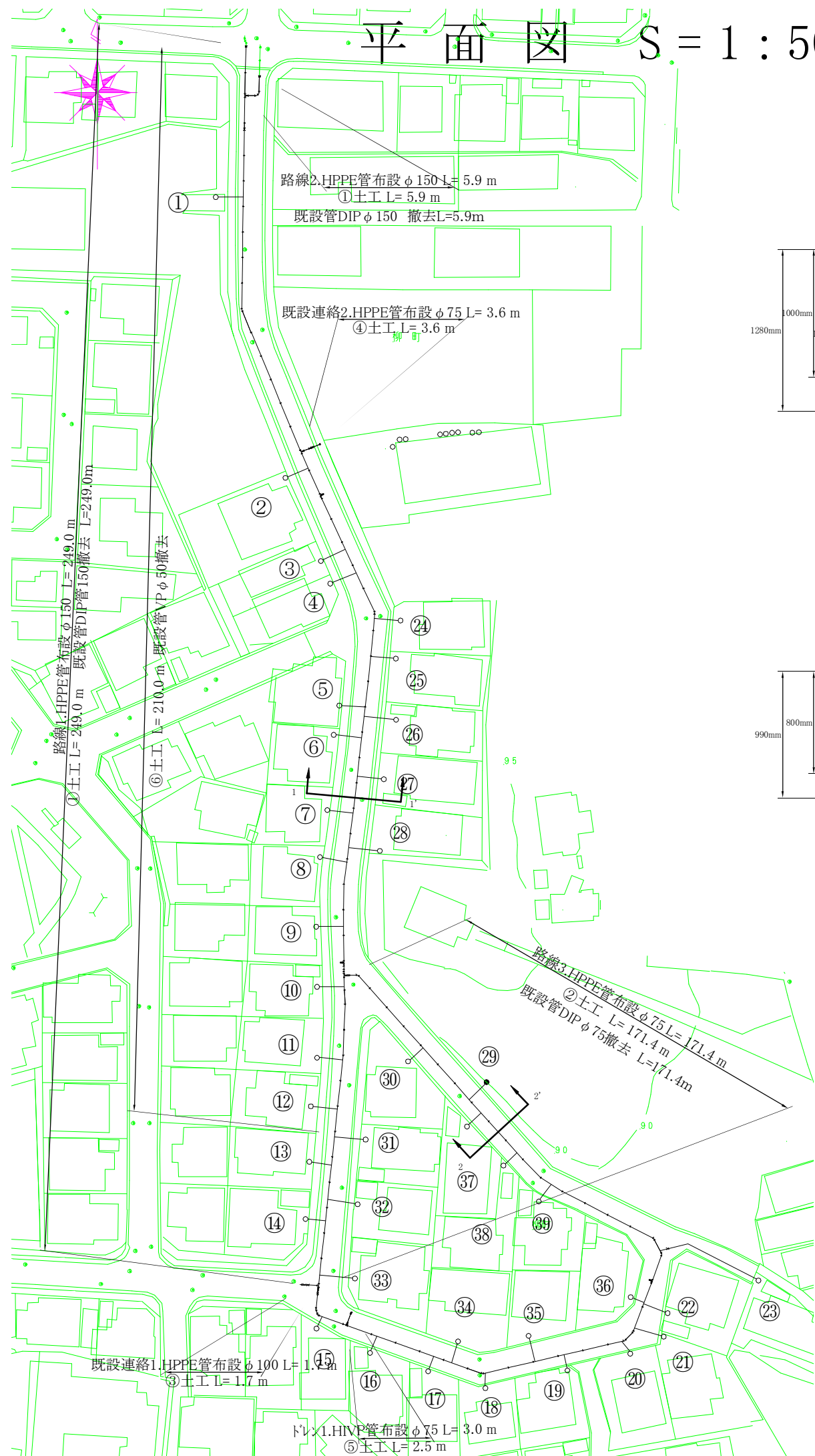
① 土工(路線1.2) HPPE管φ150布設(掘削・埋戻し) 1/20 撤去管DIPφ150
