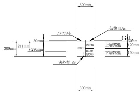
①土工(路線1、2) 仮設VLGφ75撤去 (掘削・埋戻し) 1/20
