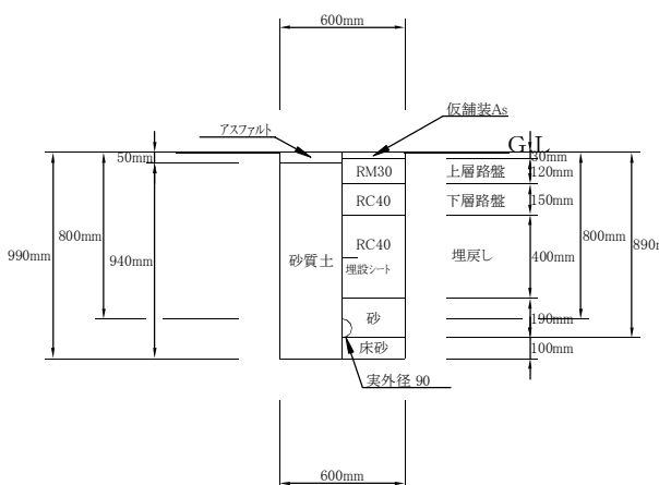
④ 土工(既設連絡2) HPPE管φ75布設(掘削・埋戻し) 1/20
