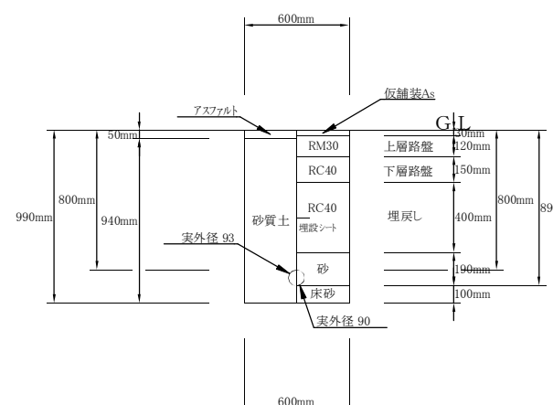
② 土工(路線3) HPPE管φ75布設(掘削・埋戻し) 1/20 撤去管 DIPφ75
