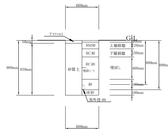
⑤ 土工(レソ) HIVP管φ75布設(掘削・埋戻し) 1/20
