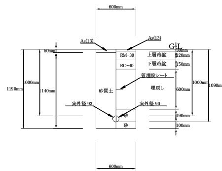
02: HPPE φ75 (掘削・埋戻し) 1/20
