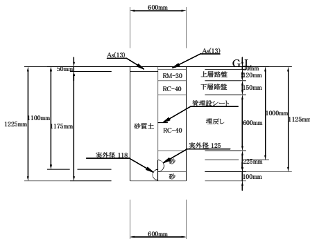
01: HPPE φ100 (掘削・埋戻し) 1/20
