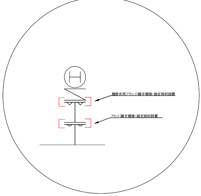
消火栓部拡大図(補強部材設置詳細)
