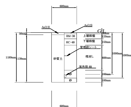
03: VP φ75 (掘削・埋戻し) 1/20
