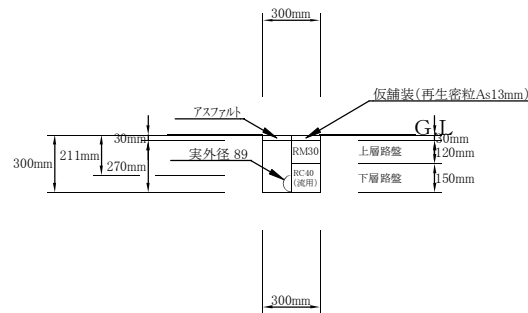
②土工 VLGφ75撤去 (掘削・埋戻し) 1/20
