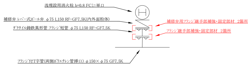
消火栓部詳細図
