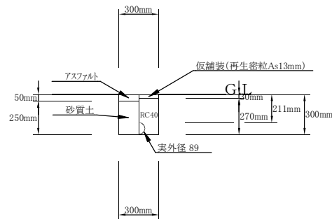
①土工 VLGφ75布設 (掘削・埋戻し) 1/20
