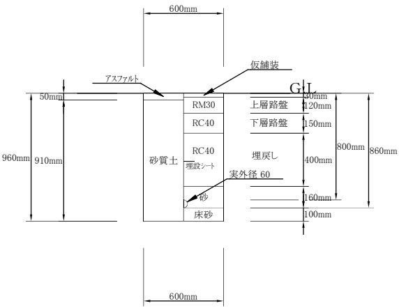
⑦土工(トレン4) HIVP管φ50布設(掘削・埋戻し) 1/20
