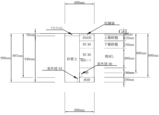
④土工(路線4、5) HPPE管φ75布設(掘削・埋戻し) 1/20 撤去DIPφ75
