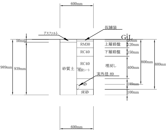
⑥土工(トレン1,2,3) HIVP管φ75布設(掘削・埋戻し) 1/20
