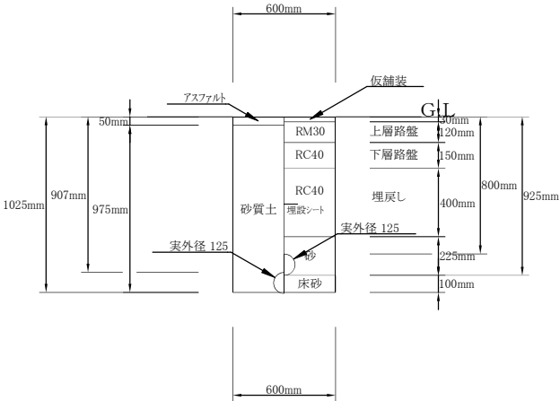
①土工(路線1、2) HPPE管φ100布設(掘削・埋戻し) 1/20 撤去DIPφ100
