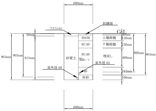
⑤土工(路線1、2) HPPE管φ50布設(掘削・埋戻し) 1/20
