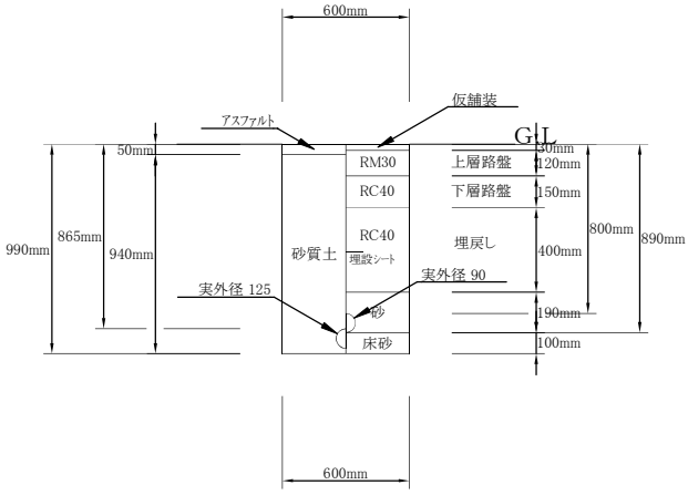
③土工(路線3、6) HPPE管φ75布設(掘削・埋戻し) 1/20 撤去DIPφ100
