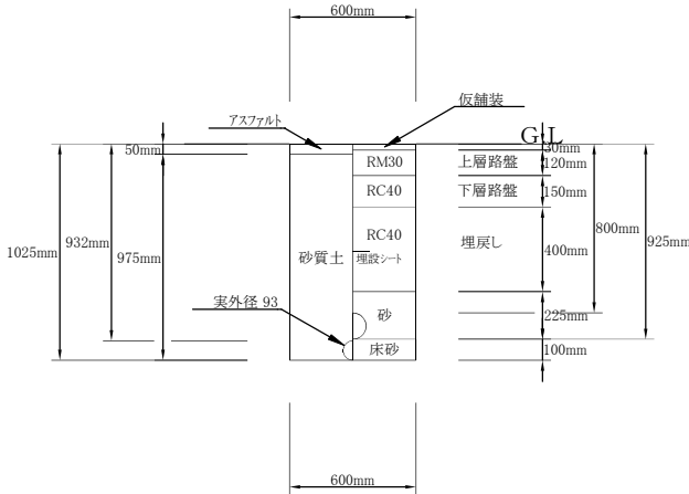
②土工(路線1) HPPE管φ100布設(掘削・埋戻し) 1/20 撤去DIPφ75
