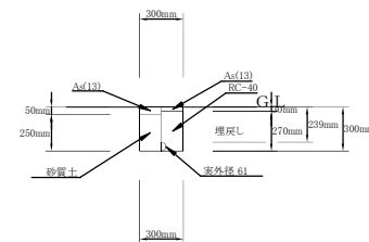
仮設 そのB 02: VLG φ50 (埋設) 1/20
