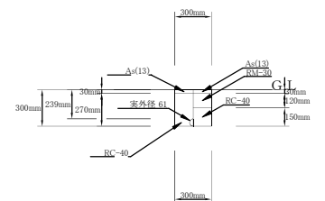
仮設 そのB 02': VLG φ50 (撤去) 1/20
