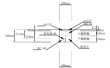
仮設 そのB 01': VLG φ75 (撤去) 1/20
