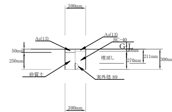
仮設 そのB 01: VLG φ75 (埋設) 1/20
