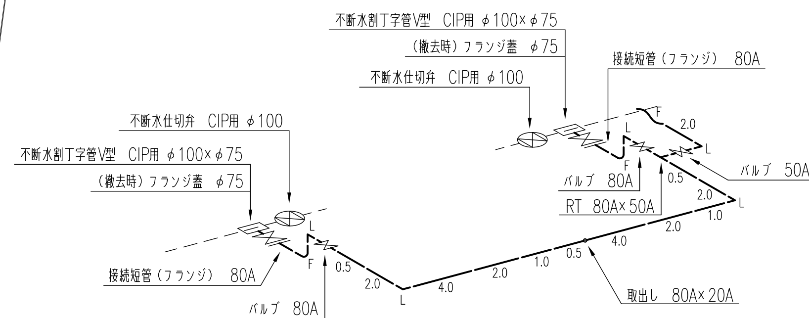
仮設配管詳細図
