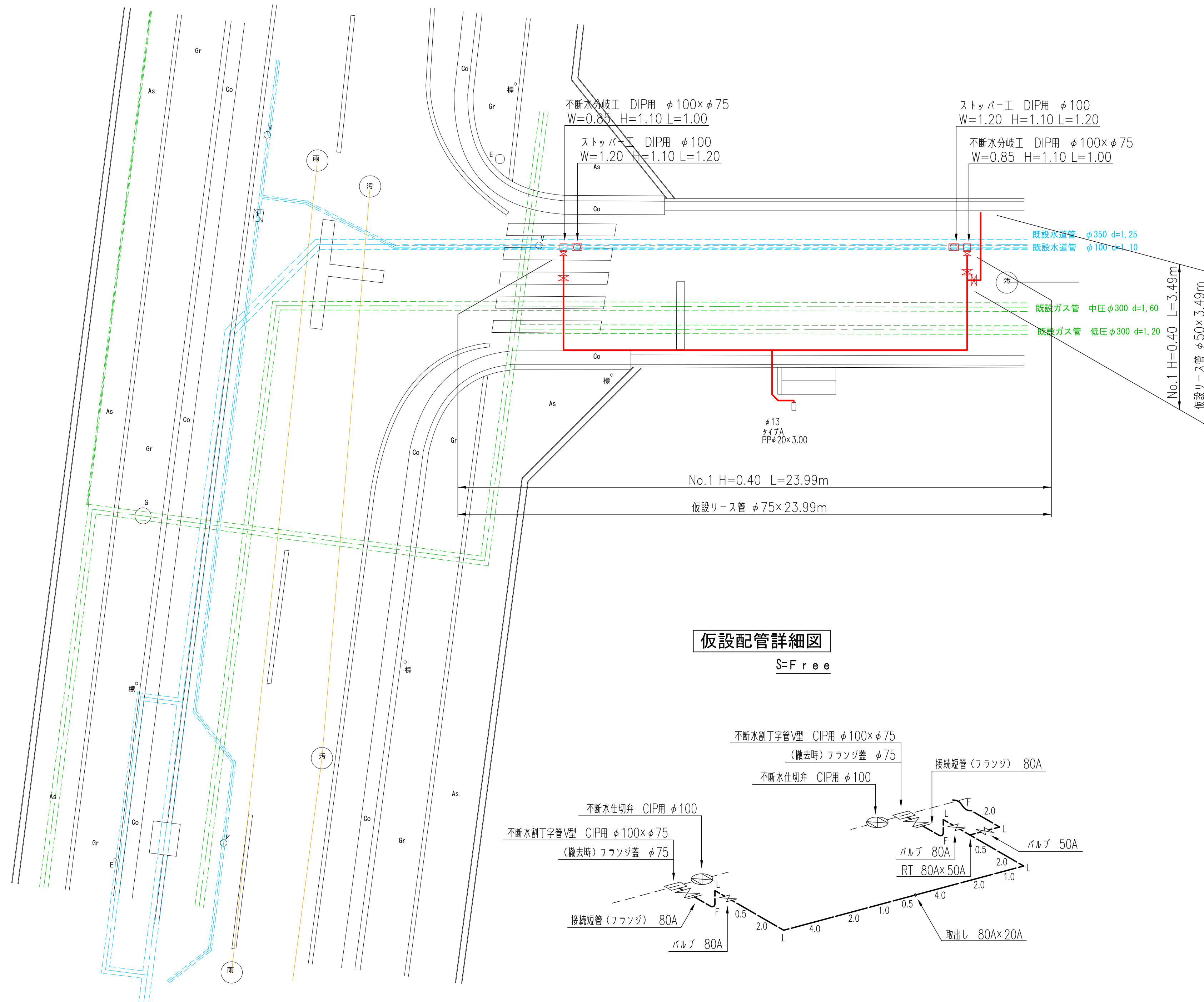
仮設配管平面図
