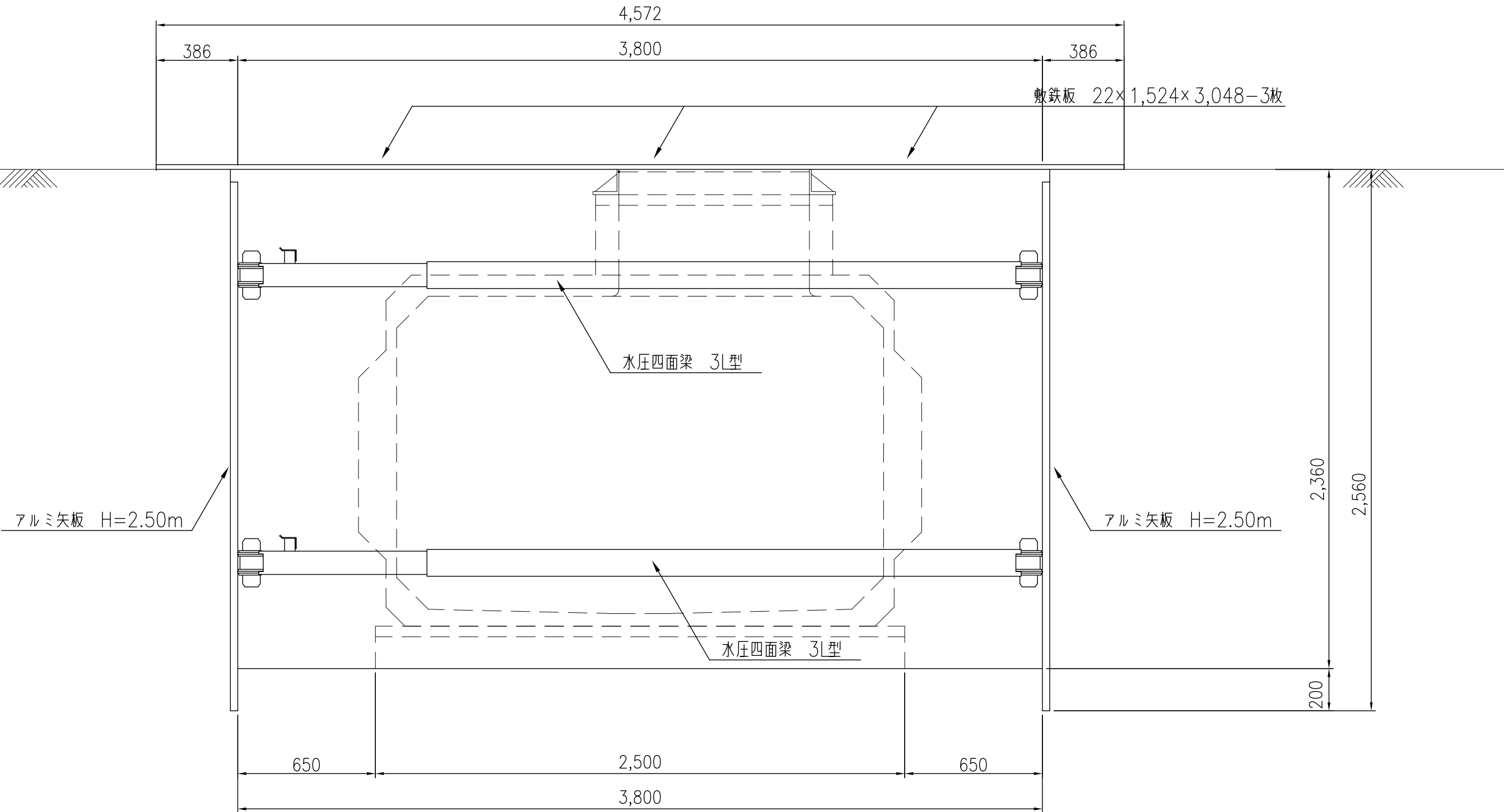
A - Ao 断面図
