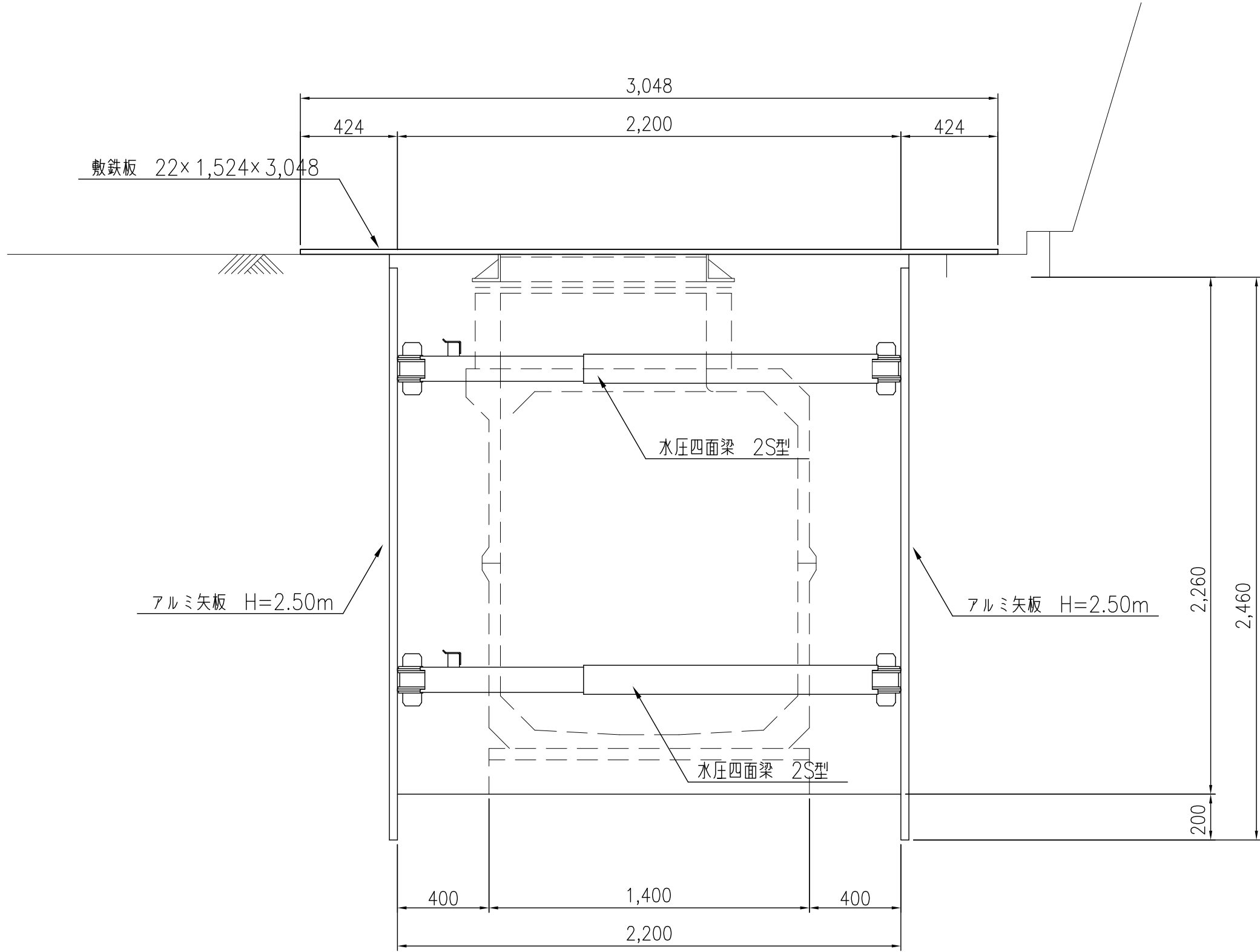
B - Bo 断面図
